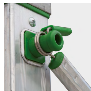
Bloqueo rápido de las diagonales con muelles en inox Bloqueio rápido das travessas diagonais com molas em inox
