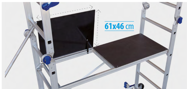
Plataforma de trabajo de tablero fenólico antideslizante con trampilla Plataforma de trabalho em placa fenólica antiderrapante com alçapão
