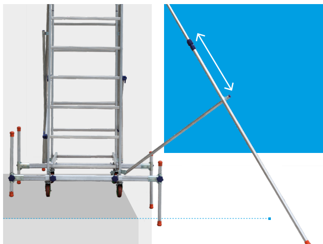
Estabilizador telescópico Estabilizador telescópico
